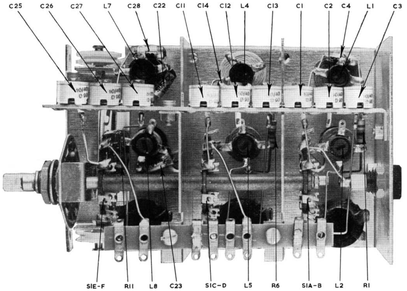
Fig. 11 R. F. chassis—European model
